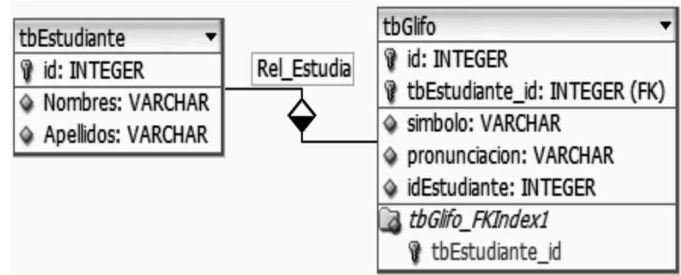
Figura 10. Vista parcial de un MER. (Software Lenguaje Maya - Edupmedia-2008 [10])
