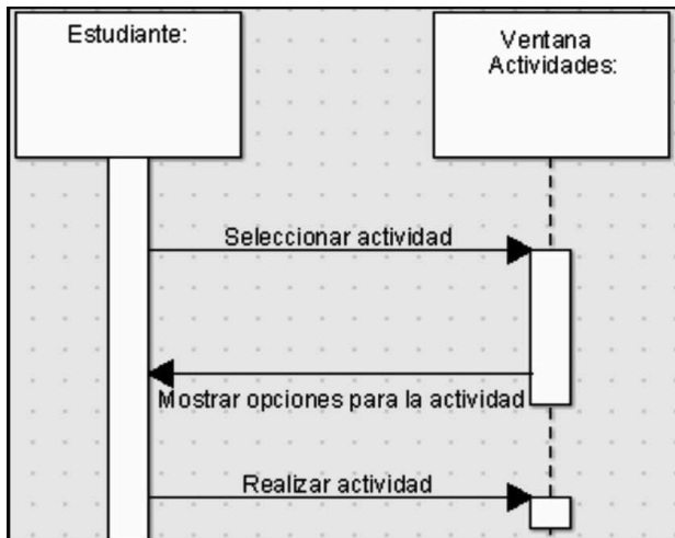
Figura 9. Ejemplo de un diagrama de secuencia. (Software Lenguaje Maya - Edupmedia-2008)
