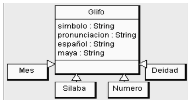
Figura 8. Ejemplo de un diagrama de clases. (Software Lenguaje Maya - Edupmedia-2008)
